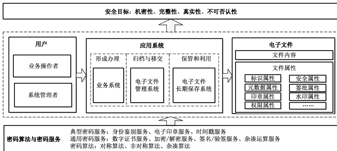
图 1 电子文件密码应用技术框架
